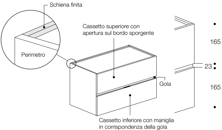
STRUTTURA CASSETTIERA
