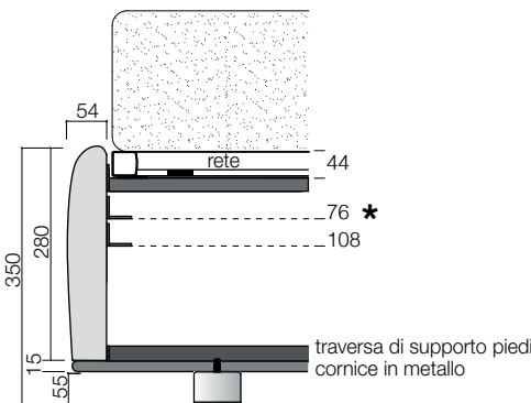
Sezione giroletto H 280 con CORNICE IN METALLO
